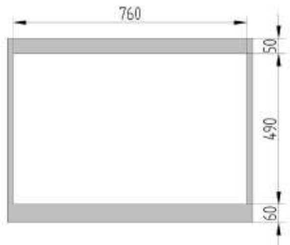
Ausschnittmaße für die Aufbaumontage
