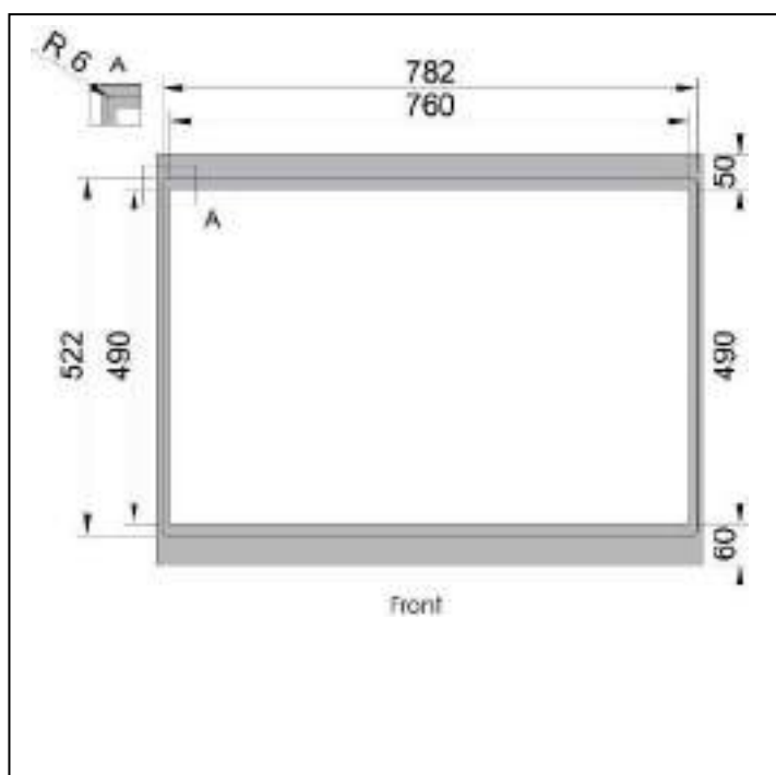
Ausschnittmaße für den flächenbündigen Einbau
